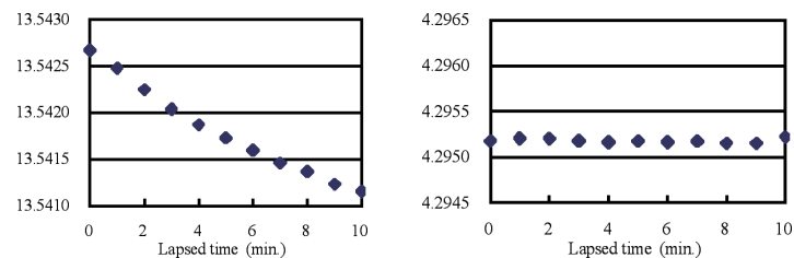
(a) 従来の表面 SH 波センサ (b) 開発した T 形表面 SH 波センサ
