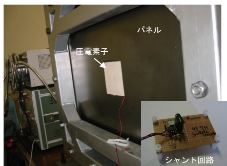
シャントダンピングシステム
