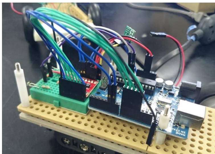
組み立てたライントレーサー
